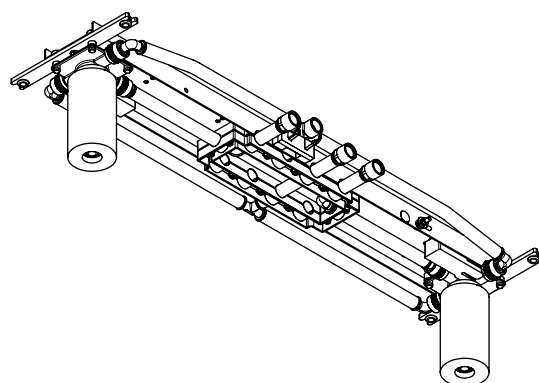
AXOR ShowerHeaven 1200 4jet 1092218X
